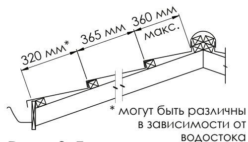
Рис. 3.5 Расположение реек обрешетки
