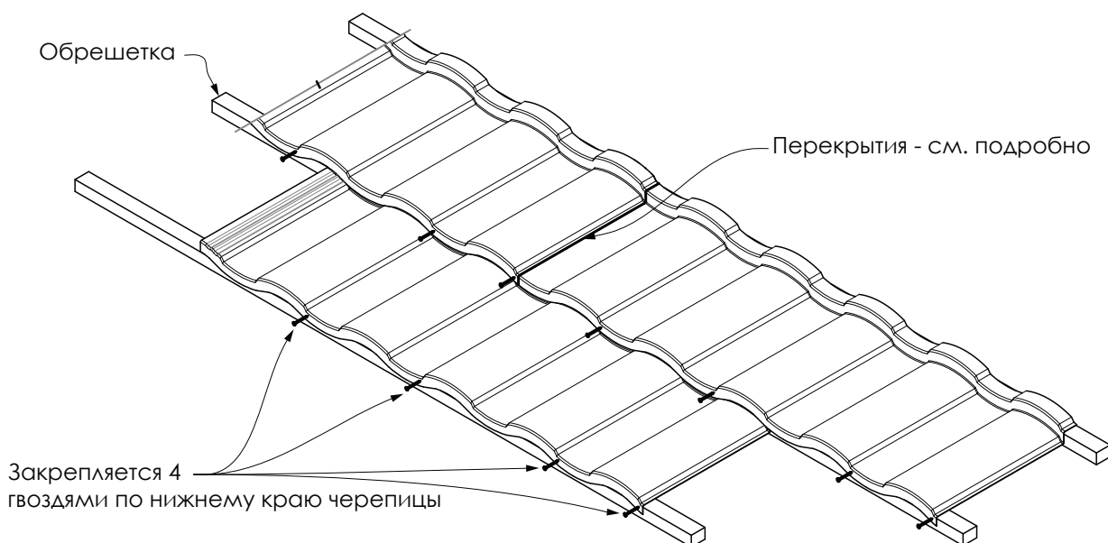
Рис. 3.2 Крепление гвоздей
