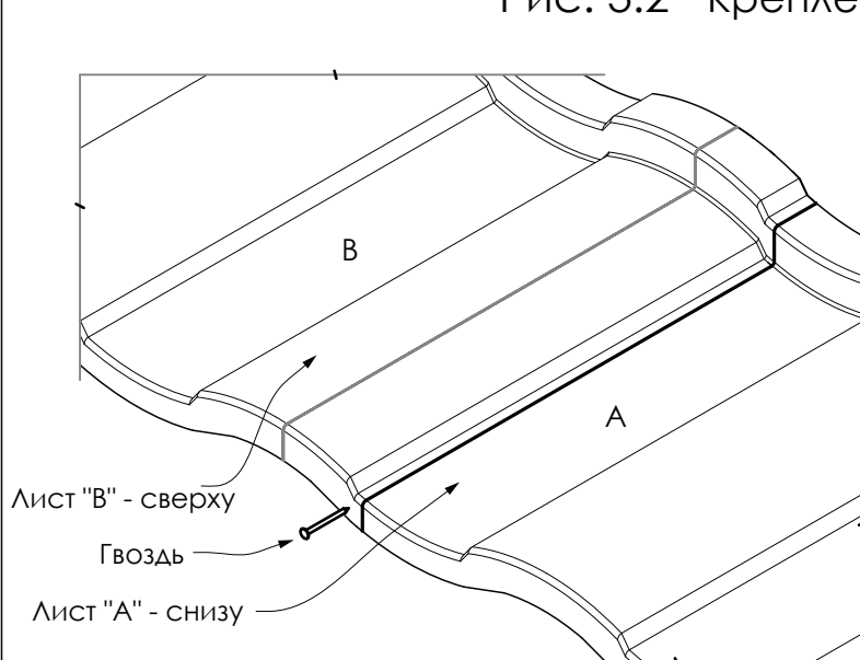
Рис. 3.3 Перекрытие листов
