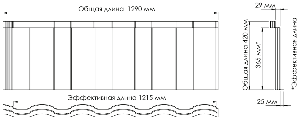
Рис. 3.1 Размеры профиля
