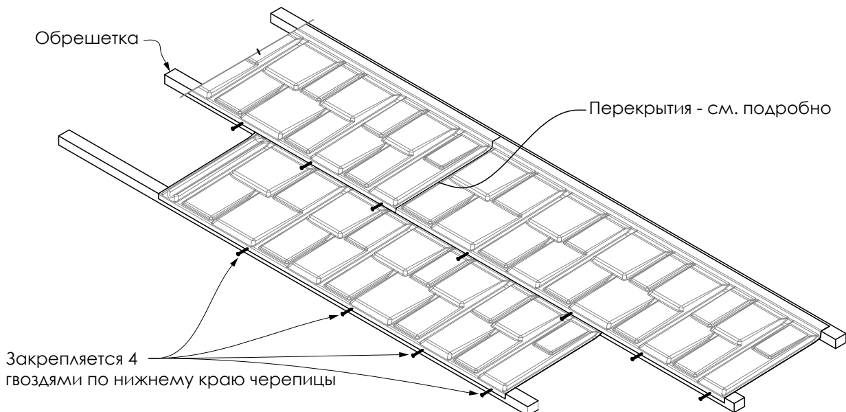
Рис. 5.2 Крепление гвоздей
