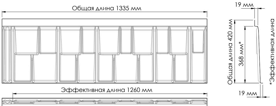
Рис. 5.1 Размеры профиля
